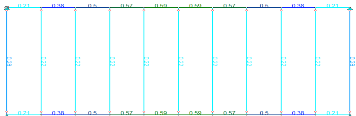
Figura 4 – Demonstração da relação do momento solicitado pelo momento resistente do aço SAE 1010 (kN.m).
