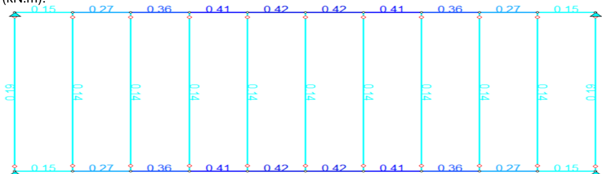
Figura 5 – Demonstração da relação do momento solicitado pelo momento resistente do USE SAC 300 (kN.m).
